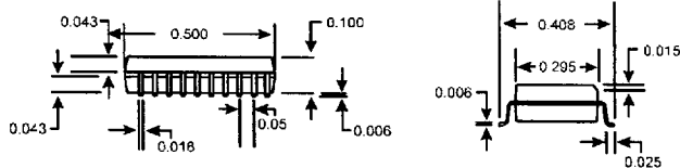
20-Pin SOIC Package
